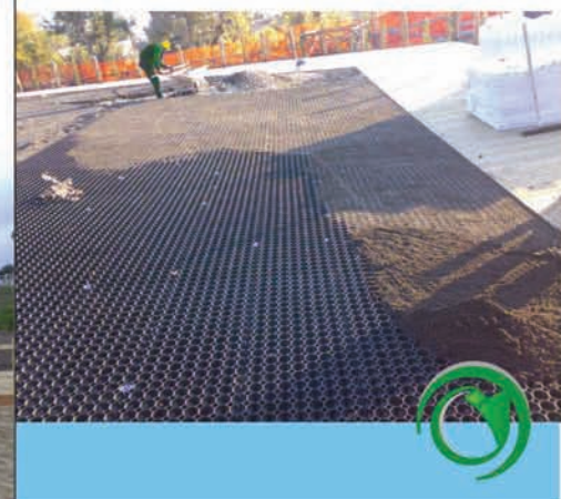
Lavori di posa in opera degli elementi in pvc riciclato per la creazione di un "prato armato" per una più sicura fruizione da parte delle persone diversamente abili
